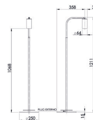
COLUNA BARI (articulada) CO 315
