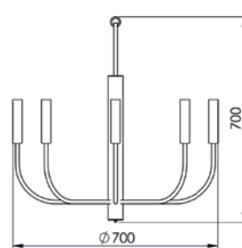
LUSTRE AMÁLIA LU 428
