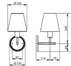
ARANDELA CORTONA AR 133
