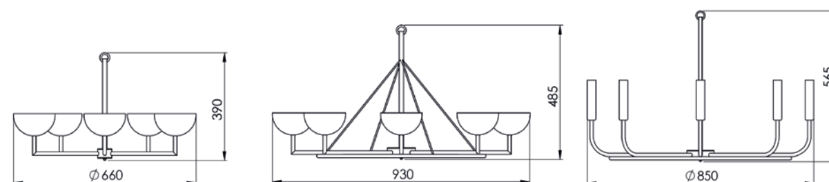
LUSTRE SAVANA 5 BRAÇOS LU 430/5
