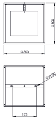
PLAFON SCATOLA PL 803
