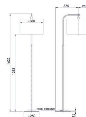
COLUNA CAPRI (articulada) CO 307
