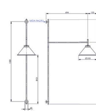
COLUNA PAREDE TORTOLI CO 321 e CO 321/LD
