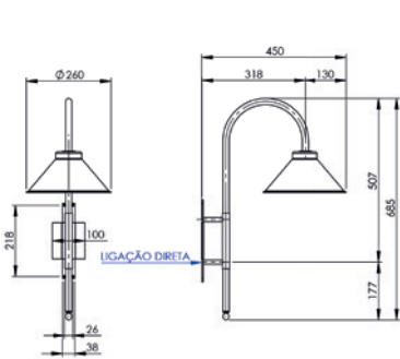
LUMINÁRIA DE JARDIM CÚPULA 26 cm J 001/26
