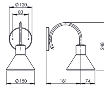
ARANDELA BIBLIOTECA AR 109
