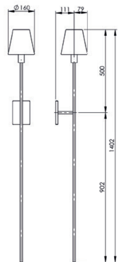
ARANDELA LUNGA QUADRADA AR 107/Q
