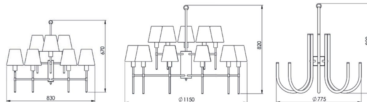
LUSTRE AMALFI 9 BRAÇOS LU 419/9
