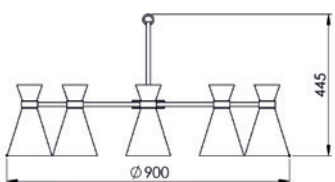
LUSTRE BELUNO 10 BRAÇOS LU 427/10
