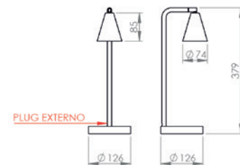
ABAJUR DANTE AB 215
