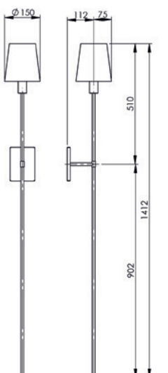
ARANDELA LUNGA AR 107/R
