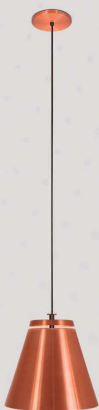
PENDENTE ORFEU 2031 Porta lâmpada: 1 x E27 Luminária: Ø 245 x 230 mm Base de teto: Ø 120 x 15 mm Cabo de alimentação: ± 2 m (regulável)
