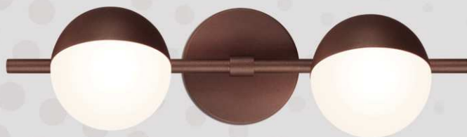
ARANDELA PALANI 1462 Porta lâmpadas: 2 x G9 Halopin Difusores: Globos de vidro branco opalino Ø 100 mm Luminária total: ⚓ 100 x ↔ 400 mm Base de parede: Ø 100 x 15 mm Profundidade: ↗ 145 mm
