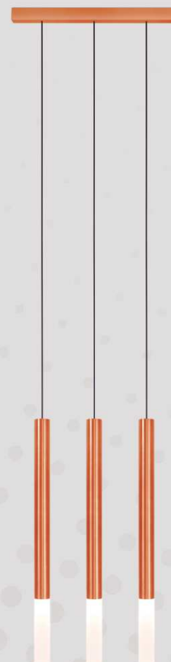
PENDENTE BILLET BRT 3 1949 Porta lâmpada: 3 x GU10 MR11 Difusores: Acrílico fosco Cada luminária: Ø 38 x Ø 530 mm Trilho de teto: 400 x 35 x 30 mm Cabo de alimentação: Ø 2 m (regulável)
