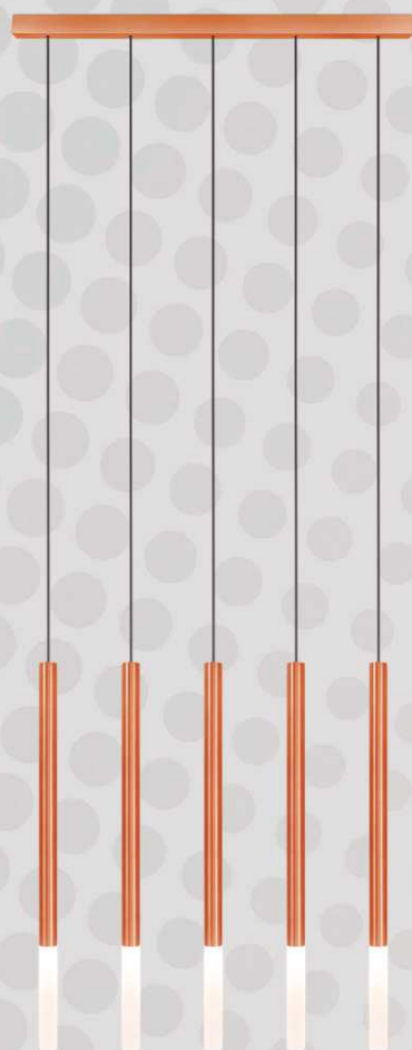
PENDENTE SLIM BILLET BRT 5 1940 Porta lâmpada: 5 x G9 Halopin Difusores: Acrílico fosco Cada luminária: Ø 25 x Ø 530 mm Trilho de teto: 500 x 35 x 30 mm Cabo de alimentação: Ø 2 m (regulável)
