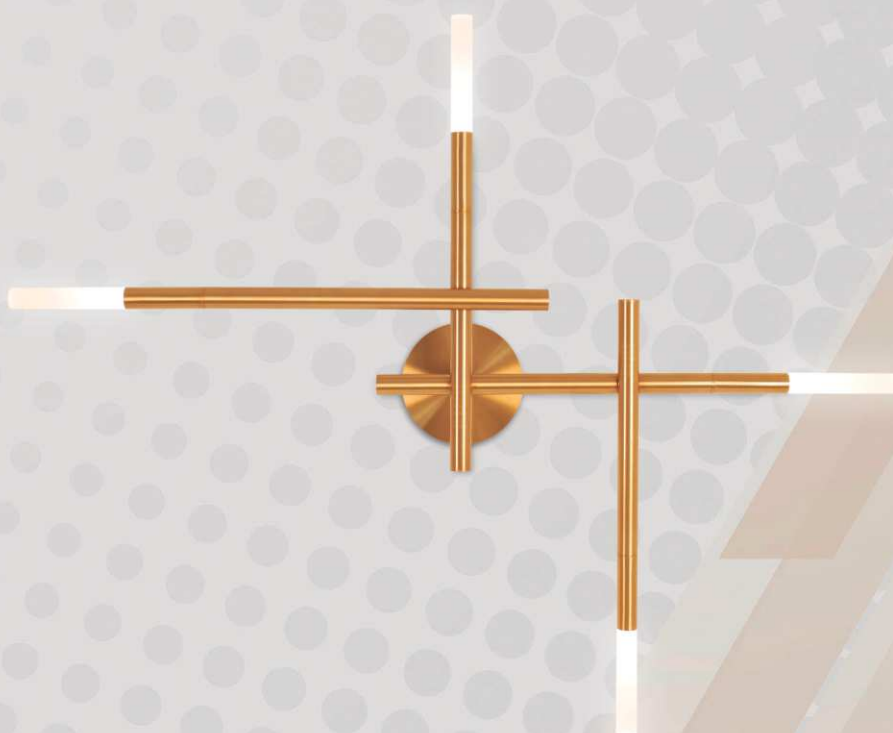
ARANDELA STEP 1691 Porta lâmpadas: 4 x G9 Halopin Difusor: Acrílico fosco Luminária total: ↔ 1040 x ∅ 840 mm Base de parede: ∅ 120 x 15 mm c/ blanquet de ∅ 150 mm Profundidade: ≥ 120 mm
