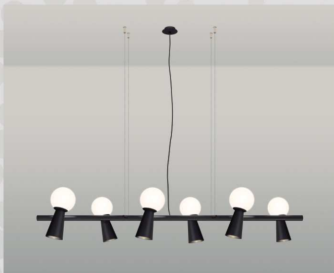
PENDENTE PION 1796 Luminária com 2 porta lâmpadas: 6 x G9 Halopin + GU10 MR16 Tamanho do spot: Ø 75mm x 120 mm
