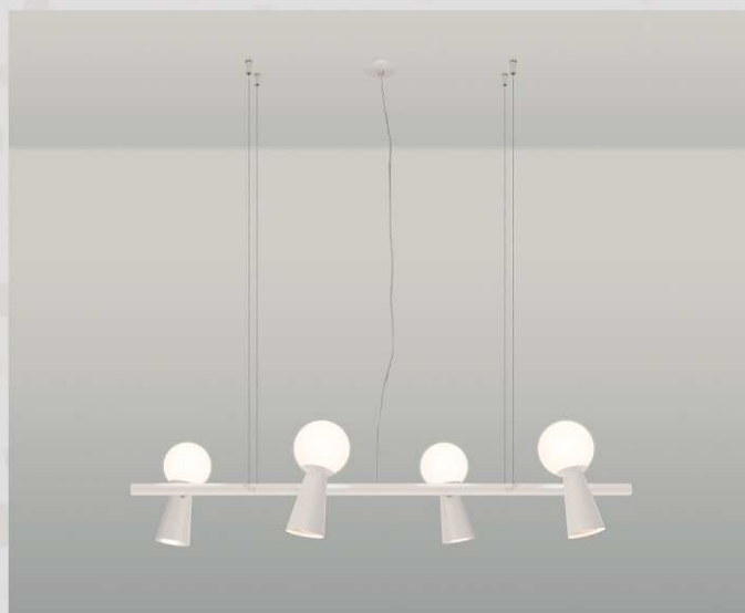
PENDENTE PION 1794 Luminária com 2 porta lâmpadas: 4 x G9 Halopin + GU10 MR16 Tamanho do spot: Ø 75mm x 120 mm
