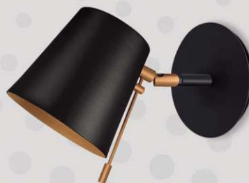
ARANDELA RAVENA POCO MOBILE 4059 Porta lâmpada: 1 x E27 Tamanho da cúpula: Ø 125 x ¢ 125 mm Luminária total: ⇔ 125 x ¢ 145 mm Base de parede: Ø 120 x 15 mm c/ blanquet de Ø 150 mm Profundidade: ≥ 175 mm
