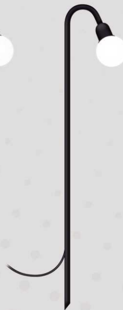
BALIZADOR SPHERA GLOBE 1349 Porta lâmpada: 1 x G9 Halopin Difusor: Globo de vidro branco opalino Ø 100 mm Luminária total: Ø 200 x ¤ 800 mm
