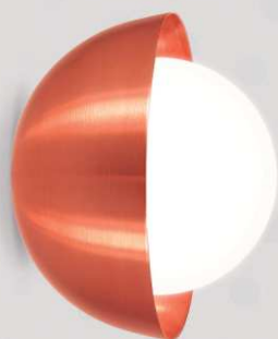
ARANDELA SUNNA 1463 Porta lâmpada: 1 x G9 Halopin Difusor: Globo de vidro branco opalino Ø 140 mm Luminária total: Ø 240 x ↔ 240 mm Base de parede: Ø 55 x 1 mm Profundidade: ↗ 170 mm
