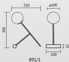
891/1 – LUMINÁRIA DE MESA IMOLA
